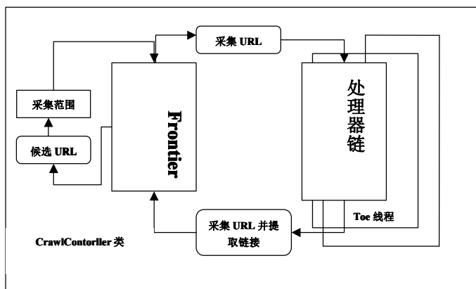
图 1.11 CrawlController 类结构
